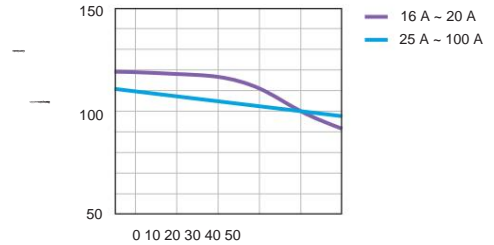
(%)Curva de reducción de temperatura ambiente
