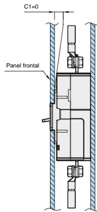
Distancia adelante/atrás en caso de panel metálico
