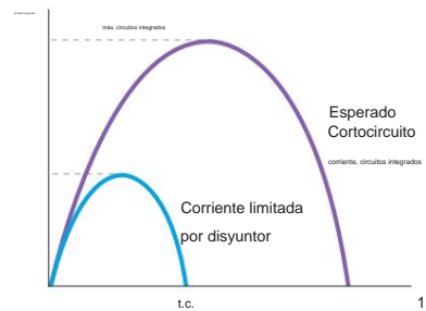
Características de limitación de corriente
