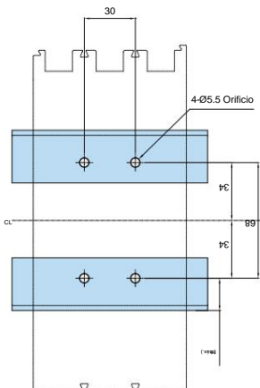
Dibujo de montaje
