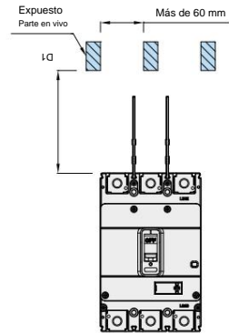
Distancia con disyuntor en caso de que la parte viva esté expuesta
