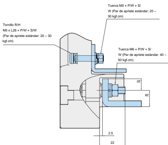
Dibujo detallado de conexión
