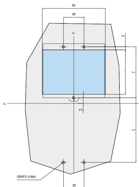
Dibujo de montaje
