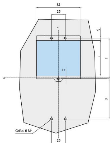
Dibujo de montaje
