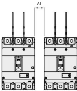
Distancia de separación en caso de que el interruptor automático se instale uno al lado del otro
