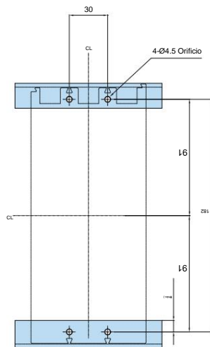
Dibujo de montaje
