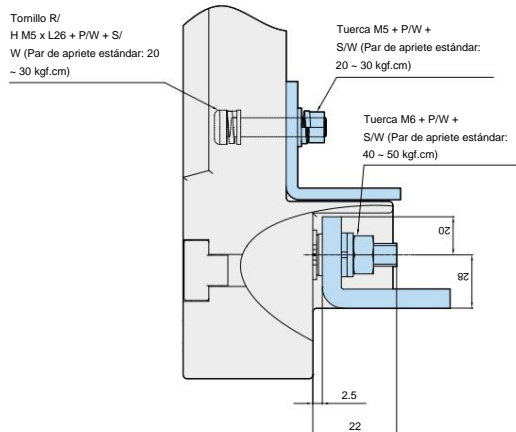
Dibujo detallado de conexión
